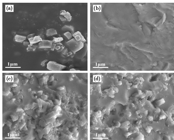
图 3 ZSM-5、SiC 和 ZSM-5/SiC 的 SEM 图
